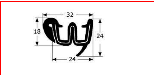
GC400 Ventanilla corredera (3,30 m)
