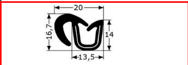
GC401 Ventanillas delanteras y traseras (2 m)
